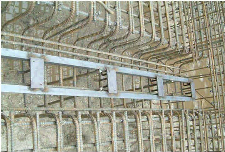
基礎錨定板安裝
