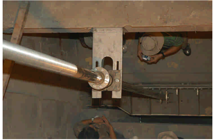
閘門吊桿安裝
